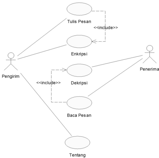
Gambar 3.4 Use Case Diagram Sistem yang diajukan.
