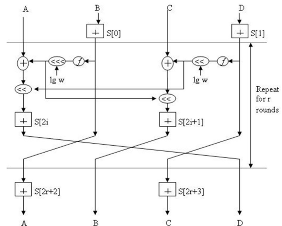
Gambar 2.1 Diagram Blok Proses Enkripsi RC 6
