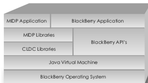
Gambar 2.3 Arsitektur sistem operasi BlackBerry (9)
