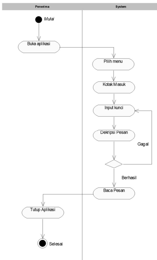
Gambar 3. 9 Rancangan Diagram Aktivitas Penerimaan Pesan Dengan Teknik Dekripsi
