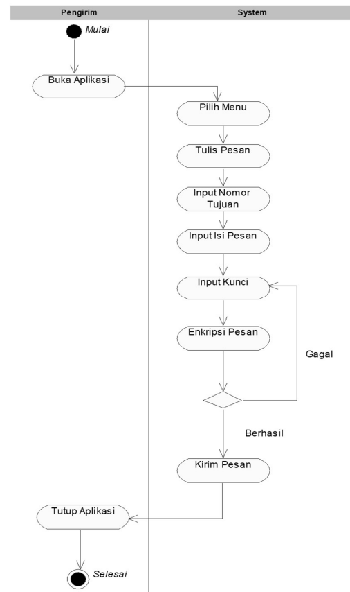
Gambar 3.8 Rancangan Diagram Aktivitas Pengiriman Pesan Dengan Teknik Enkripsi
